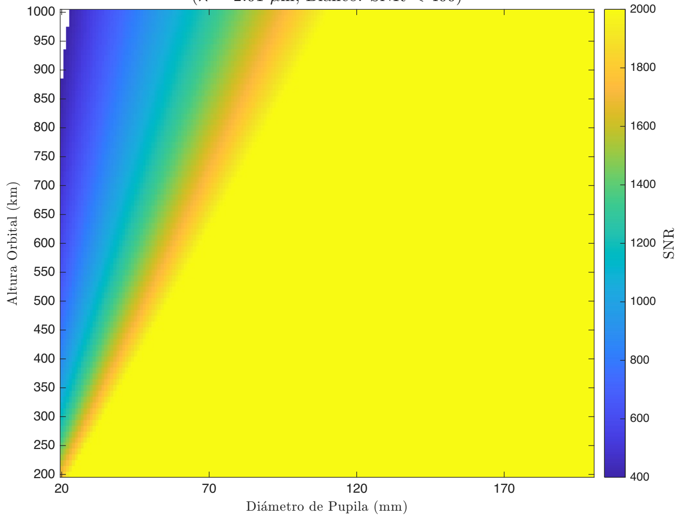
SNR - Korsch - Detector 3 ( \lambda = 2.01 \mu\text{m} , Blanco: SNR < 400)
